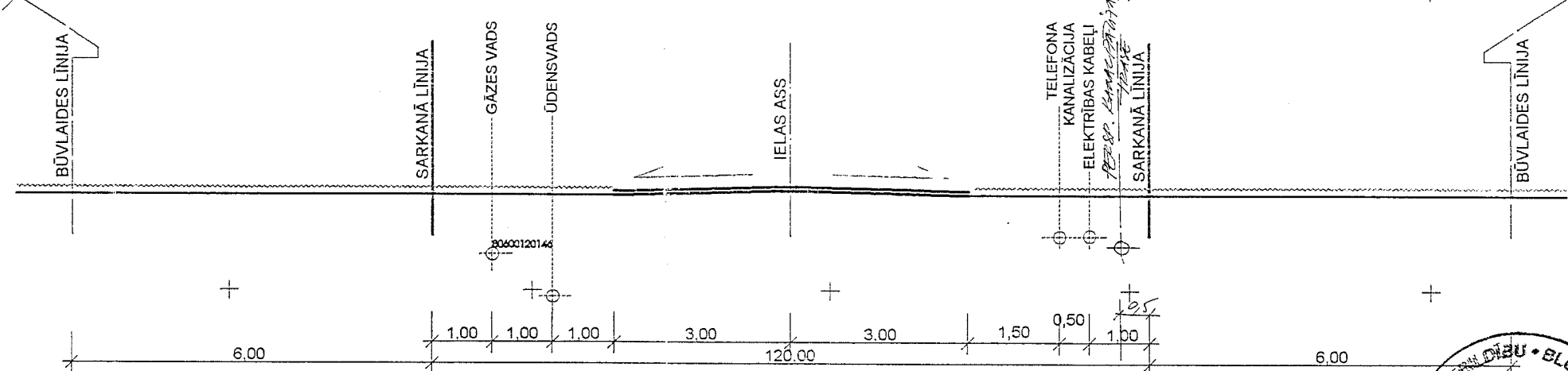
IELAS PROFILS B-B M 1:100
