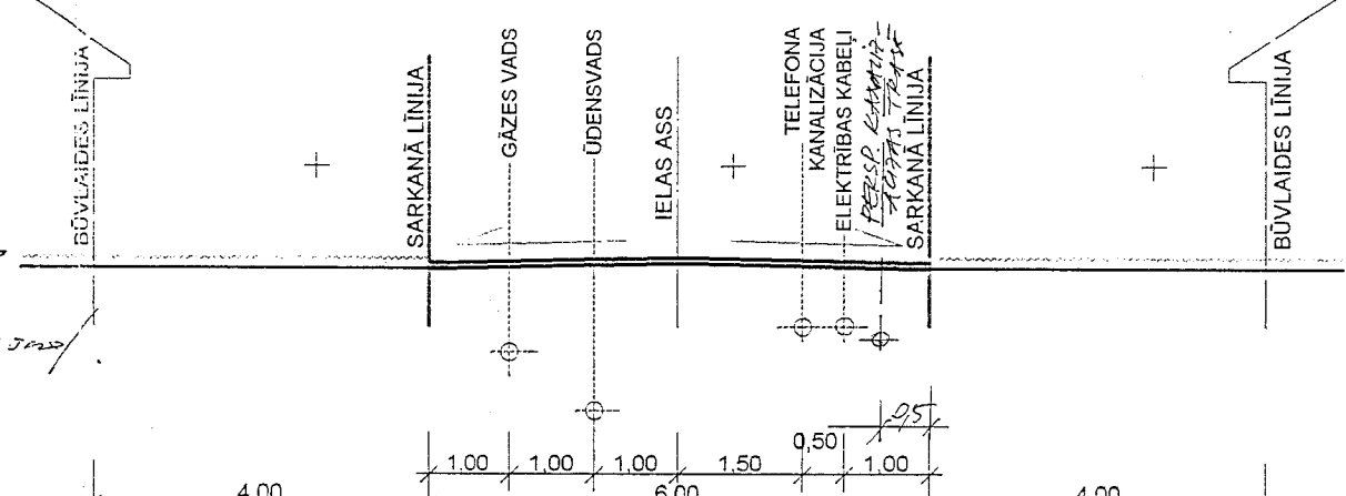
IELAS PROFILS A-A M 1:100
